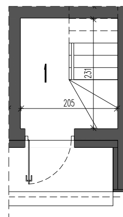
RZUT PARTERU
