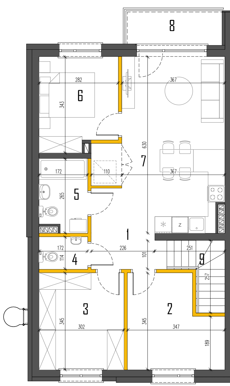
RZUT PIĘTRA
