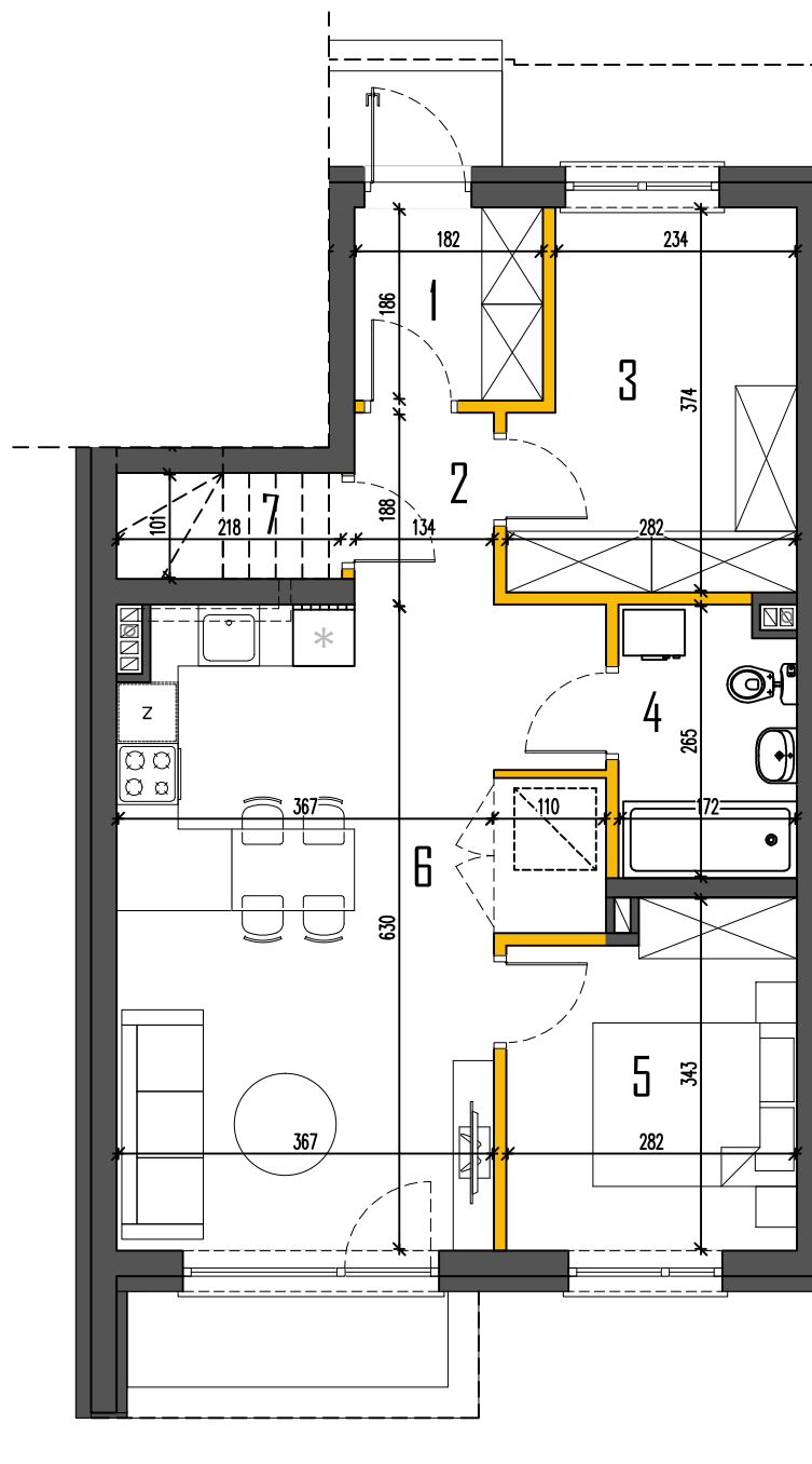
RZUT PARTERU
