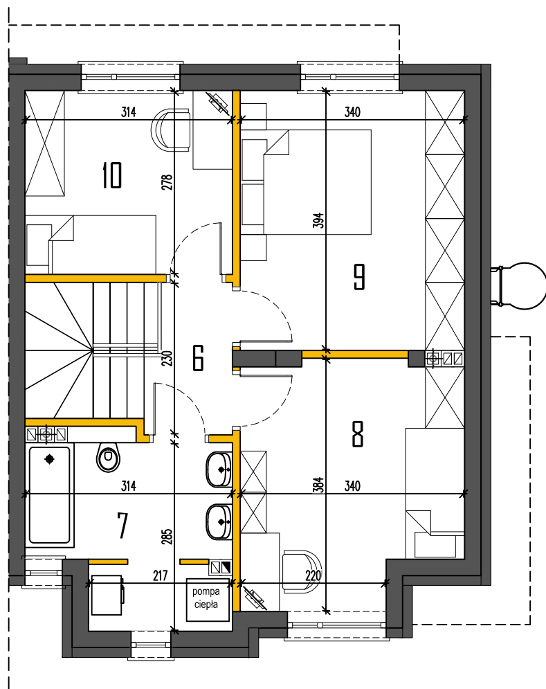
RZUT PIĘTRA
