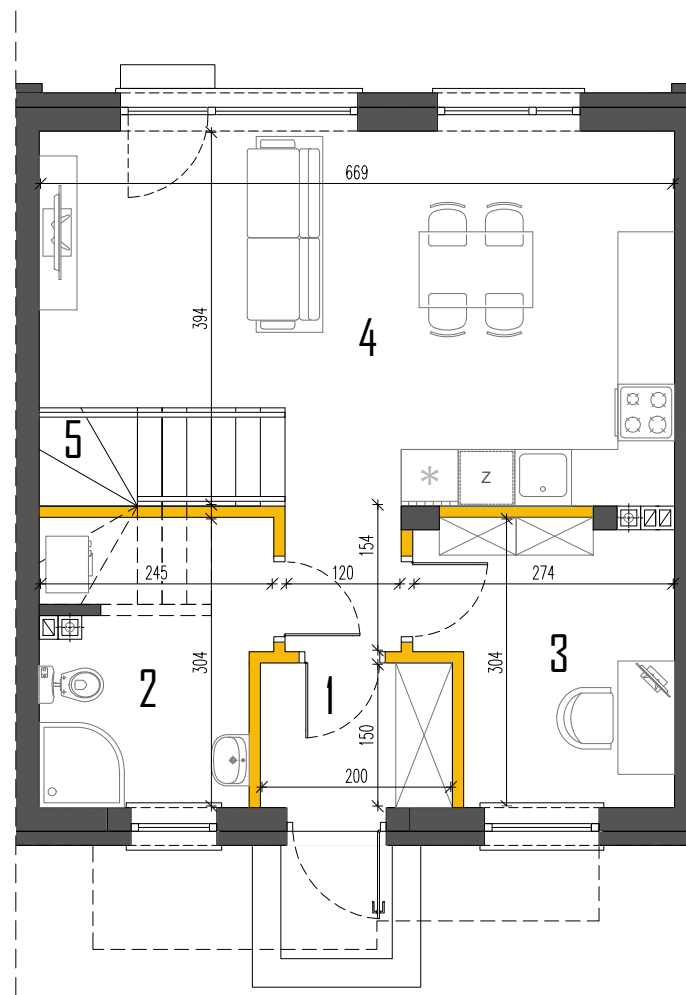
RZUT PARTERU
