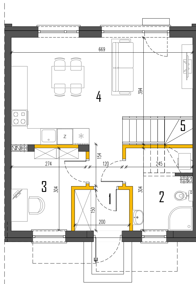
RZUT PARTERU
