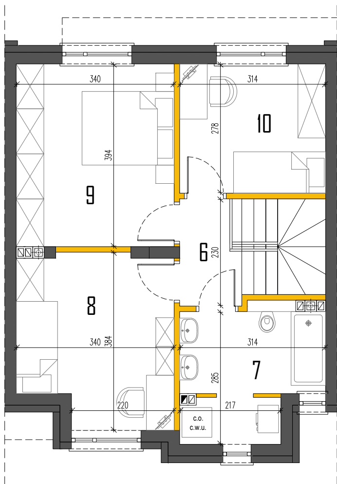
RZUT PIĘTRA
