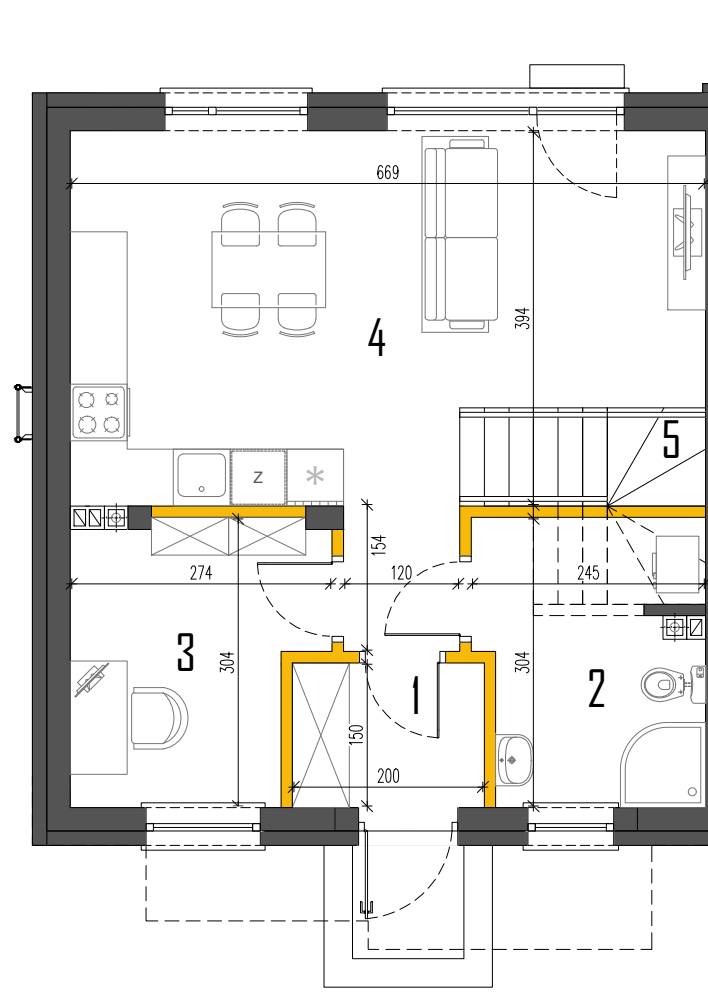
RZUT PARTERU
