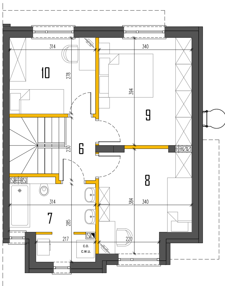
RZUT PIĘTRA
