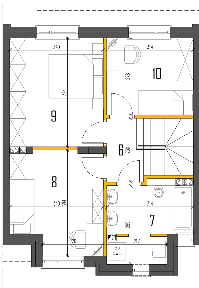
RZUT PIĘTRA
