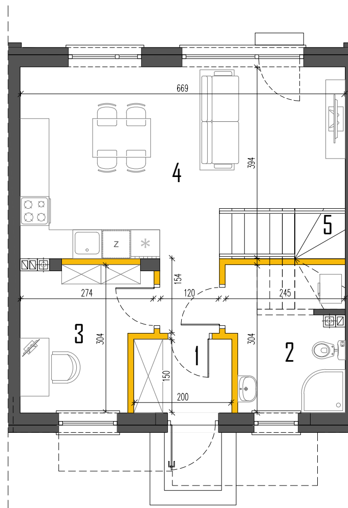
RZUT PARTERU
