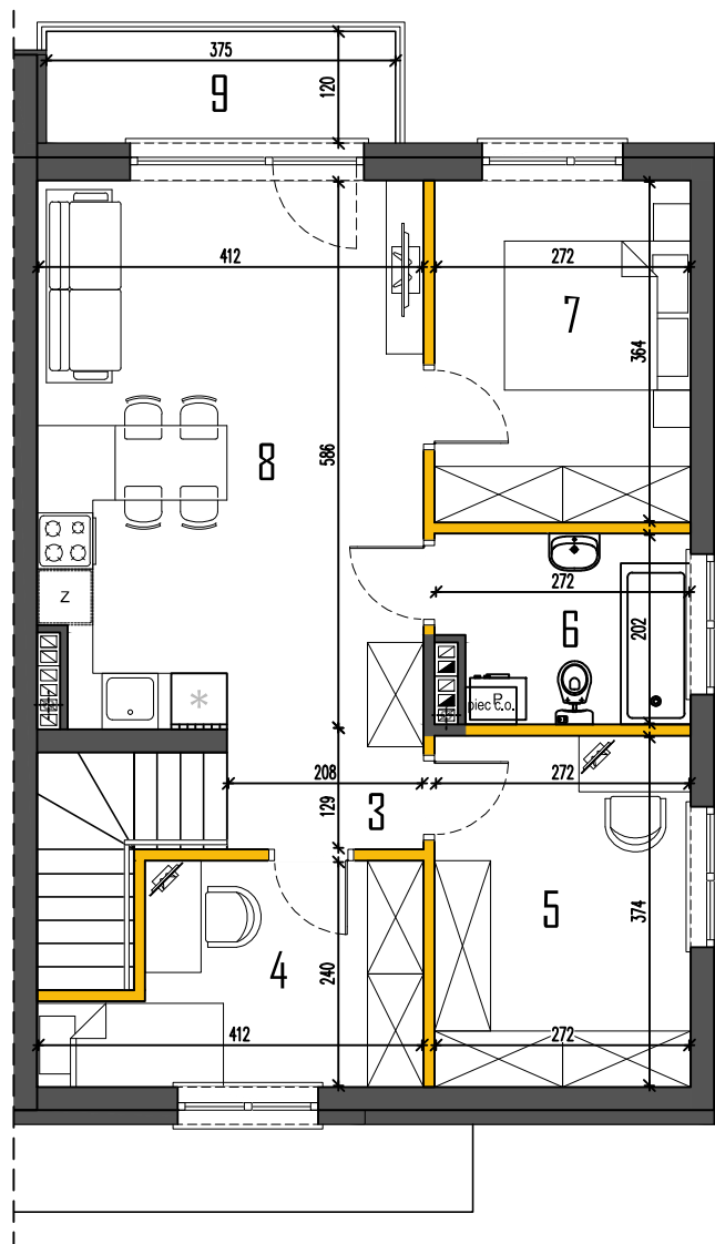
RZUT PIĘTRA
