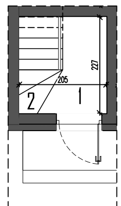
RZUT PARTERU
