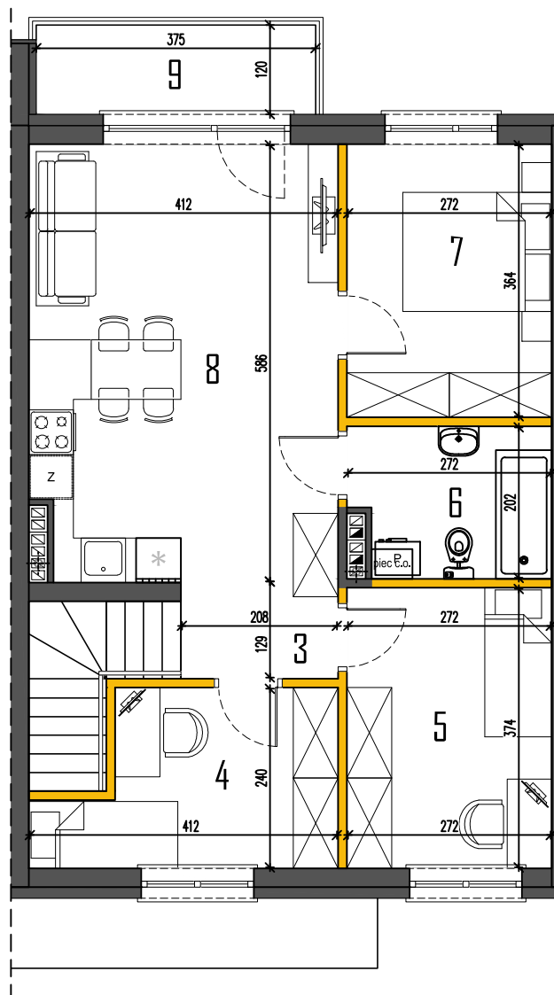
RZUT PIĘTRA
