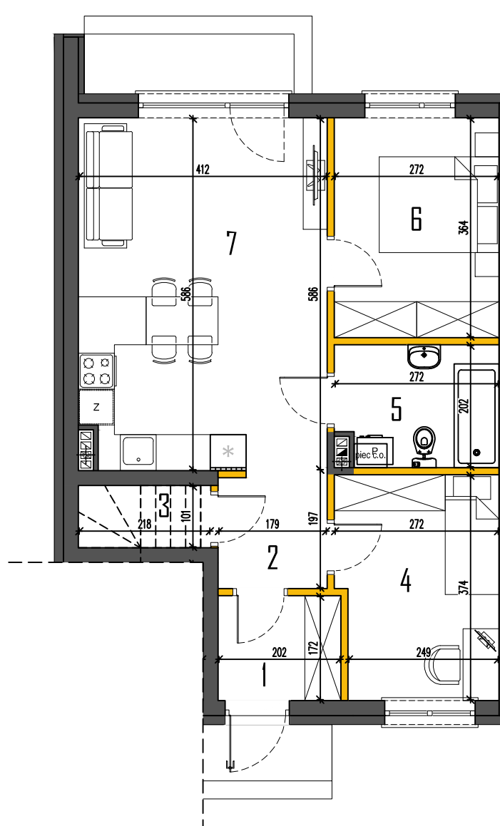
RZUT PARTERU
