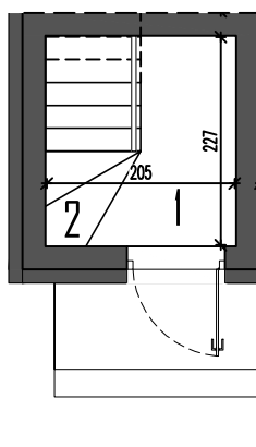
RZUT PARTERU
