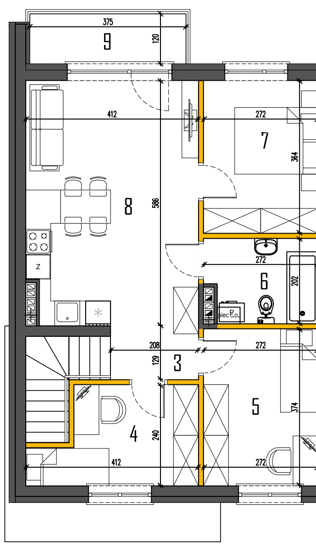
RZUT PIĘTRA
